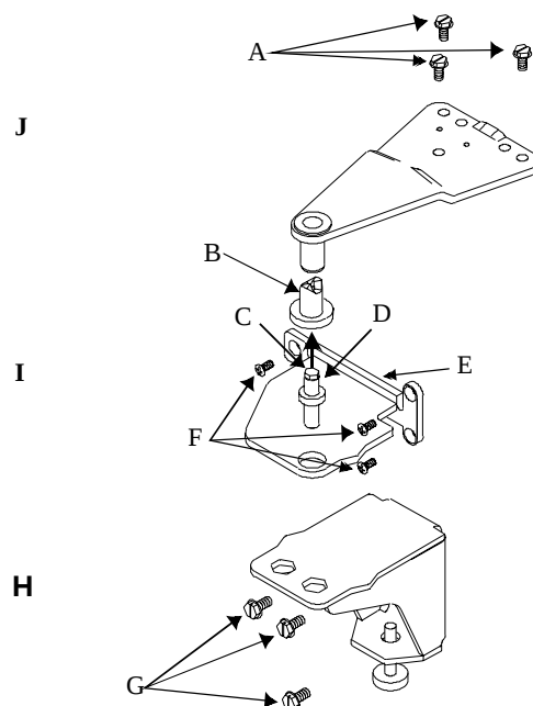
A. Vis de 5/16 po (8 mm) B. Ferme-porte C. Écrou hexagonal de 5/16 po (8 mm) D. Axe de la charnière centrale E. Support de la charnière F. Vis cruciformes G. Vis de 3/8 po (10 mm) H. Charnière inférieure I. Charnière centrale J. Charnière supérieure
